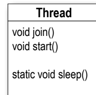
java.lang.Thread class
